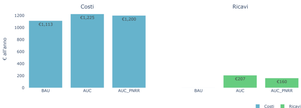
Costi e ricavi per scenario - utente consumer
