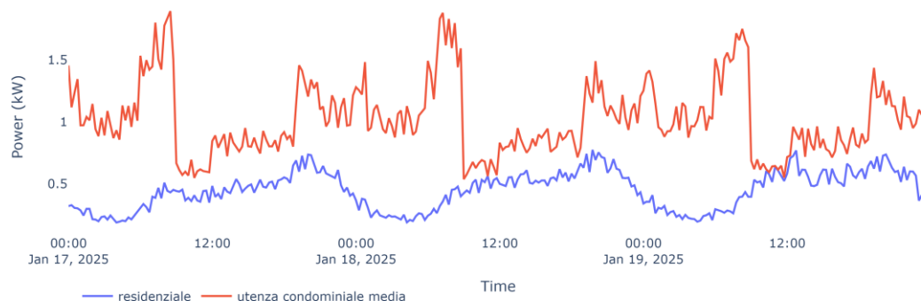
Esempio curve di carico di tre giorni (giorno ferial, sabato e domenica)
