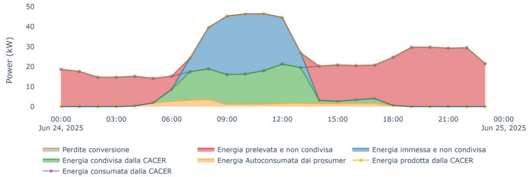
Flussi energetici - 2025-06-24 - CACER
