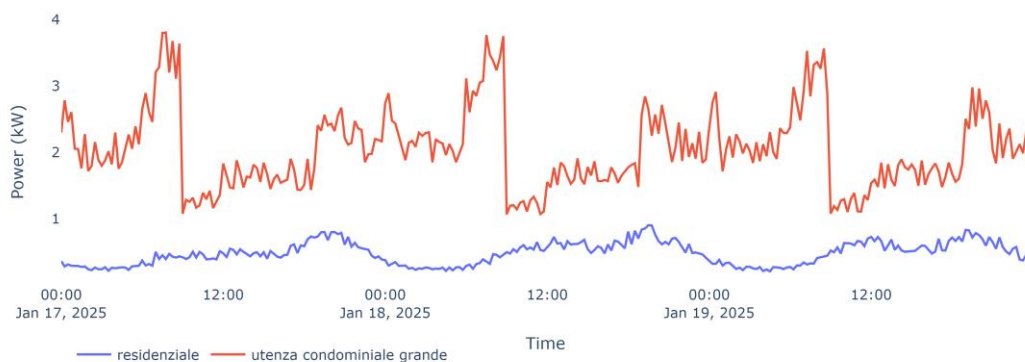
Esempio curve di carico di tre giorni (giorno ferial, sabato e domenica)
